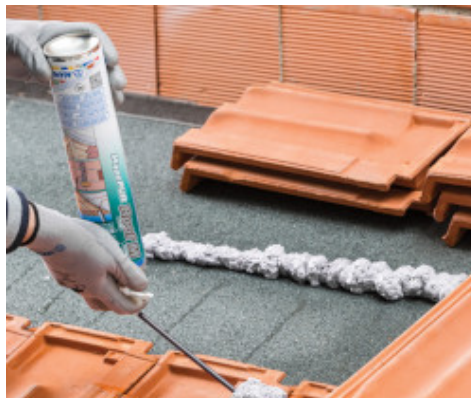
Punktweise Verklebung von Dachziegeln
